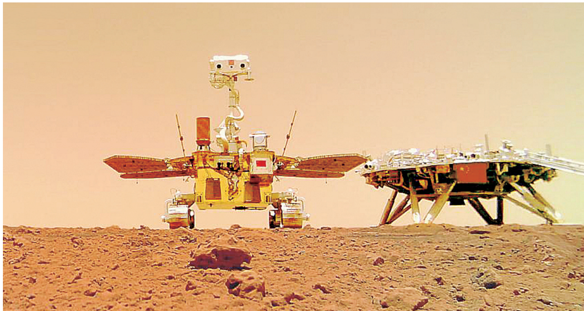
2021年6月11日,国家航天局在北京举行天问一号探测器着陆火星首批科学影像图揭幕仪式,公布了由祝融号火星车拍摄的着陆点全景、火星地形地貌、“中国印迹”和“着巡合影”等影像图。这是“着巡合影”图。 国家航天局供图
