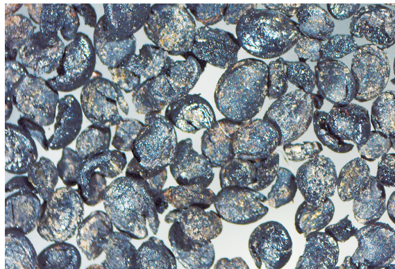
鸽子山遗址出土的浮选植物种子。
